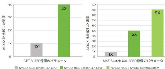
GPT-3のAI学習を最大9倍高速化
